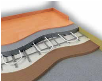
IZOLACIJA TAL PRI TALNEM OGREVANJU
